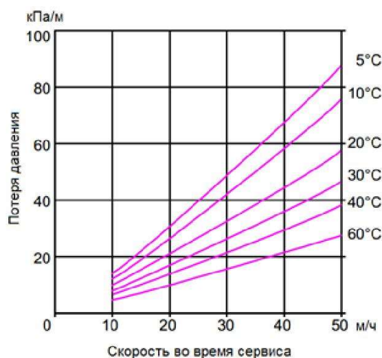
Рис. 2. Потери давления
