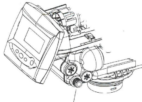
Место подключения реагентной трубки
